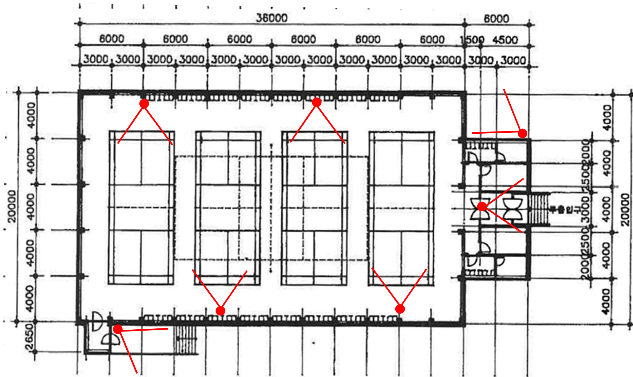
1층 평면도 S: 1/300
